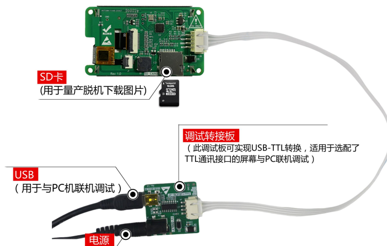
图 1-5 调试工具图
