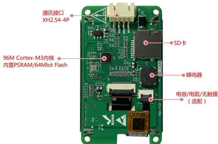
图 1-4 硬件配置图
